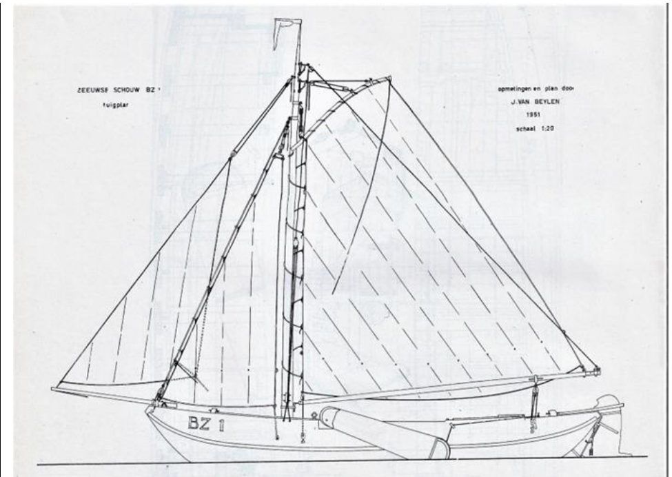
Afb. 30. J. VAN BEYLEN, tuigplan van een Zeeuwse schouw naar opmetingen van een origineel, 1952. Antwerpen, Nationaal Scheepvaartmuseum, nr. A.S. 54.56.1.
