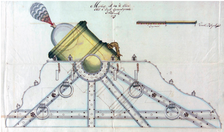
Mortier voor kogels of granaten tot 100 pond als krombaangeschut in stelling.
